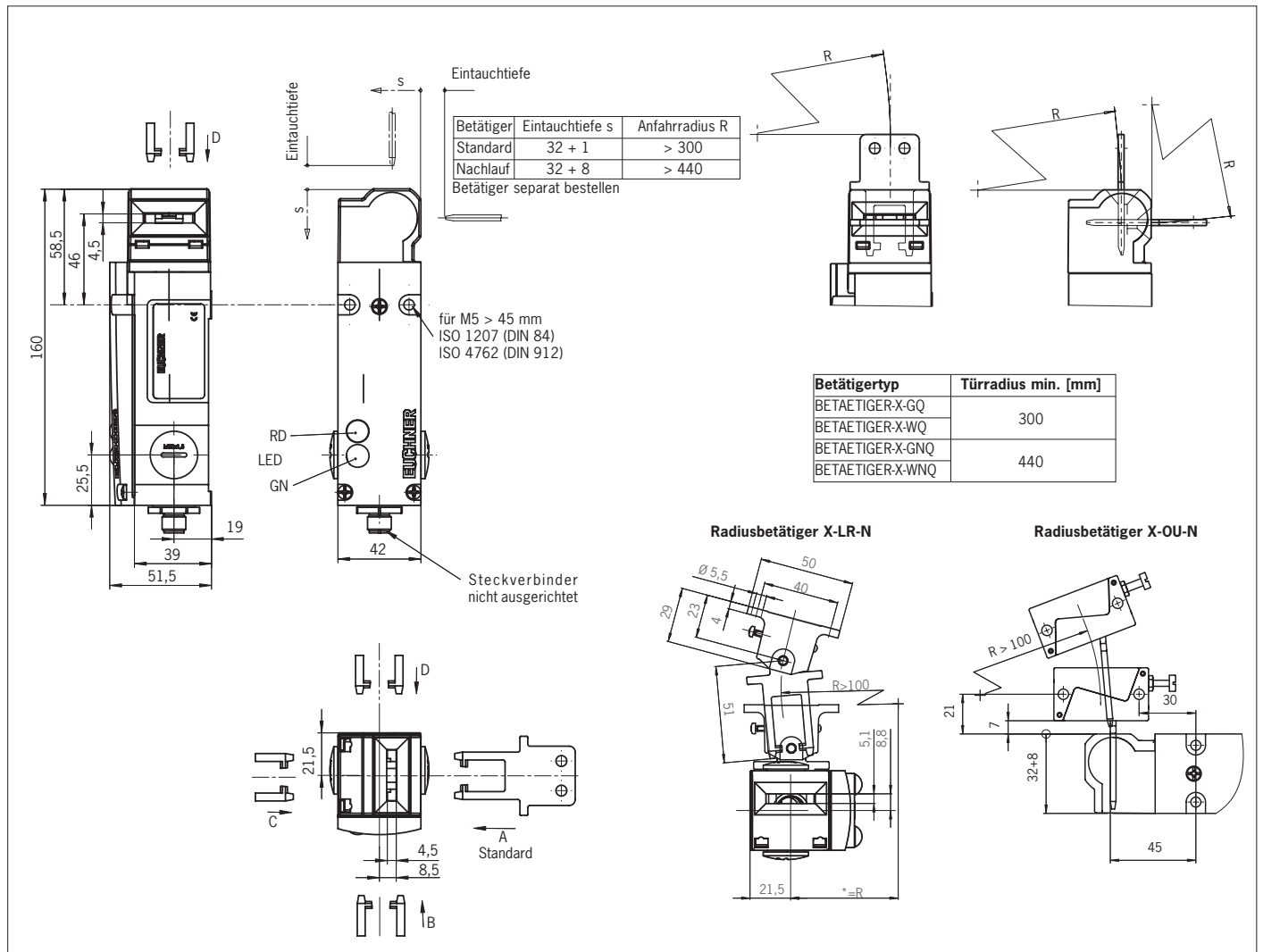
Bild 4: Maßzeichnung NX...AS1, Eintauchtiefe und Anfahradien
