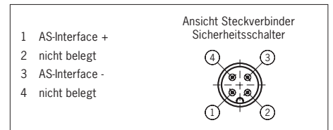
Bild 3: Anschlussbelegung AS-Interface M12-Steckverbinder
