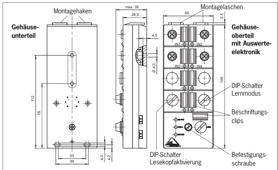
Bild 2: Maßzeichnung CES...AS1 (Abbildung zeigt Ausführung CES-AF1B-04B-AS1)
