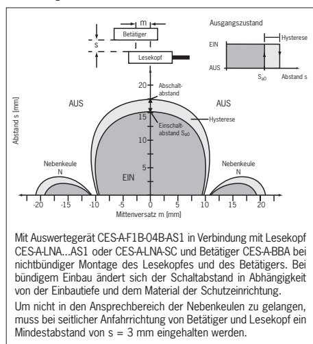
Bild 3: Typischer Ansprechbereich
