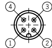
Ansicht Steckverbinder Notaus-Schaltgerät
